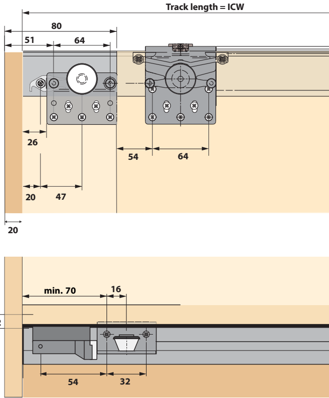
Abbreviations : DW - Door Width / ICW - Internal Cabinet Width / DH - Door Height / TH - Total Height
